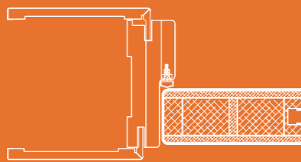
Конструкция дверного блока в сборе
